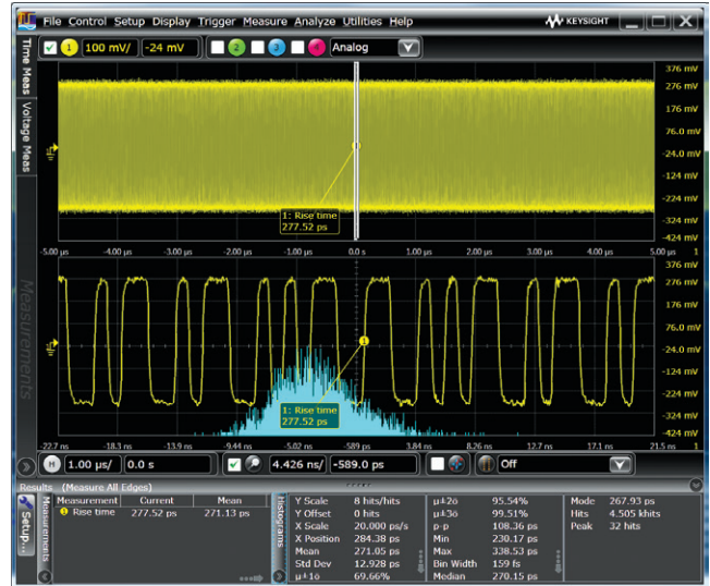
그림 39. InfiniiView는 다양한 고급 신호 분석 기능은 물론, 광범위하고 직관적인 파형 문서화 기능을 제공합니다.
