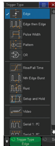
그림 42. 다양한 고급 파라메트릭 트리거 모드
