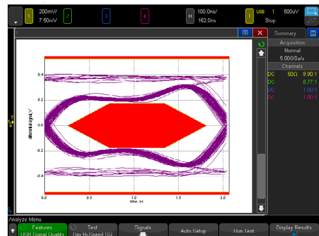
그림 27. USB 2.0 저속, 최고 속도 및 고속 신호에 대한 자동 신호 품질 테스트를 수행합니다.
