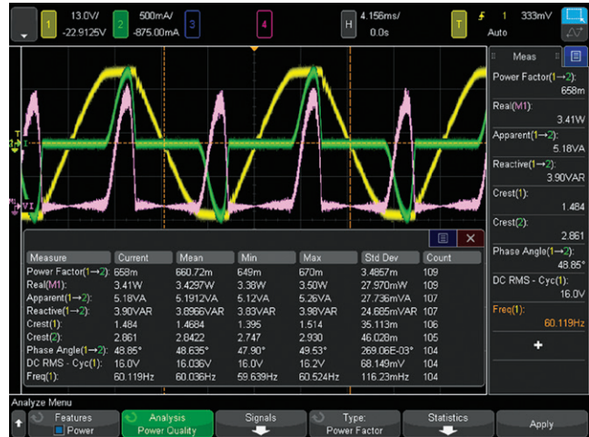
그림 25. 전력 품질 측정, 많은 전력 측정 어플리케이션 중 하나
