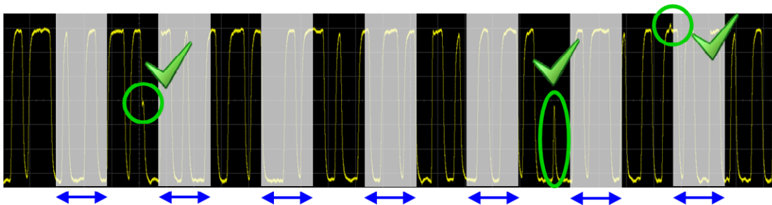
그림 5. 초당 100만 파형 속도의 InfiniiVision 4000 X-시리즈. 짧은 데드타임은 간헐적 이벤트를 수집할 수 있는 확률을 높입니다.
