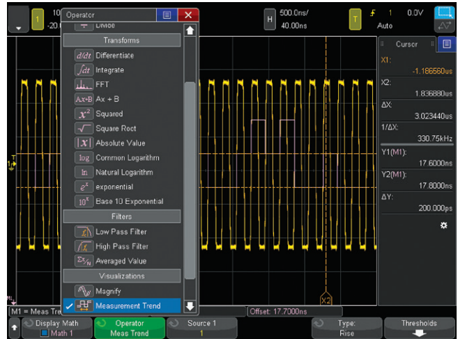
그림 30. 4000 X-시리즈에는 다양한 고급 수학 함수가 기본적으로 들어 있습니다.
