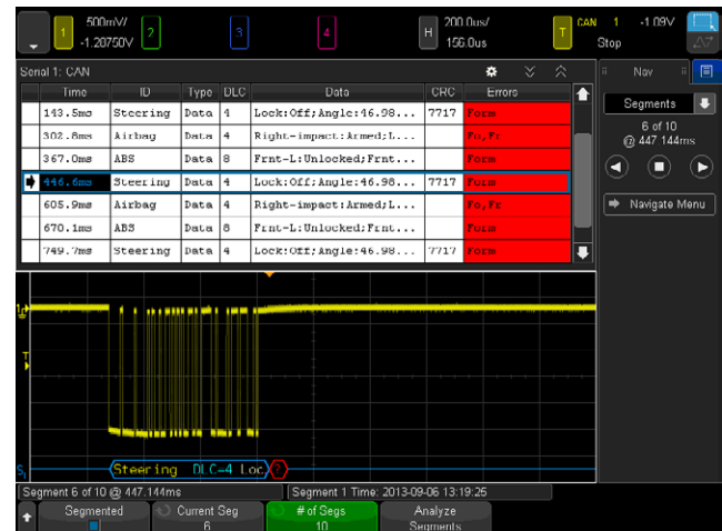
그림 8. 세그먼트 메모리 및 시리얼 디코드의 결합으로 시리얼 버스에 대한 통찰력을 극대화합니다.
