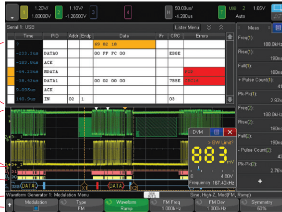
그림 17. 4000 X-시리즈는 5가지 계측기 기능이 매끄럽게 하나로 통합되어 있습니다.
