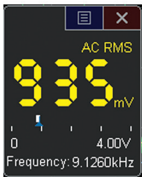
그림 24. DVM 3 디지털 전압 및 5 디지털 주파수 측정은 언제든지 손쉽게 이용할 수 있습니다.
