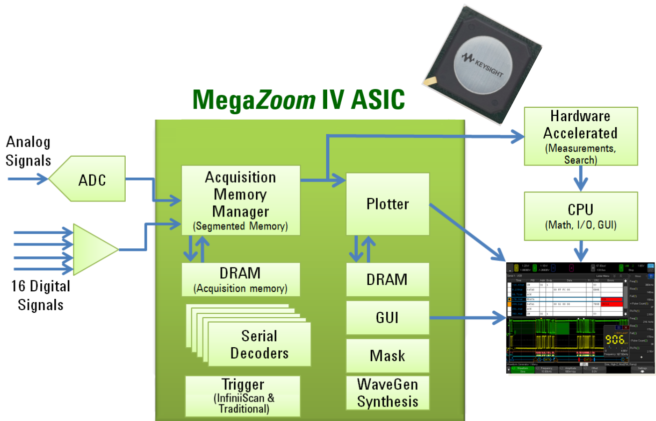
그림 6. 4000 X-시리즈 오실로스코프는 MegaZoom IV, 스마트 메모리 ASIC를 통해 매우 빠른 응답성, 속도 및 파형 업데이트 속도를 제공합니다. 주요 파형 작동시 CPU가 사용되지 않습니다.
