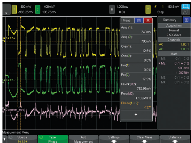
그림 23. 차동 임의 신호의 듀얼 채널 WaveGen 출력. 공통 모드는 수학적 함수로 표시됩니다.
