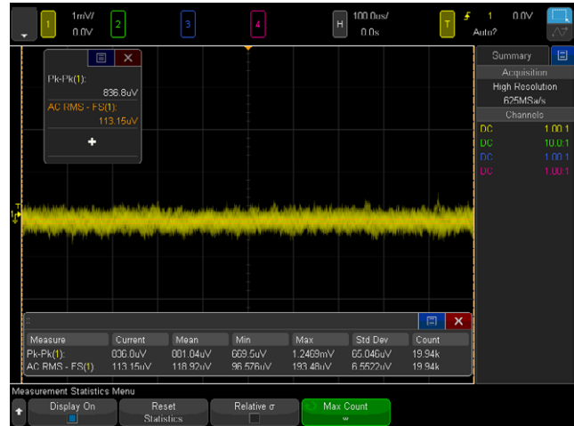
그림 41. 고분해능 모드로 최대 12비트까지 수직 분해능을 높입니다.
