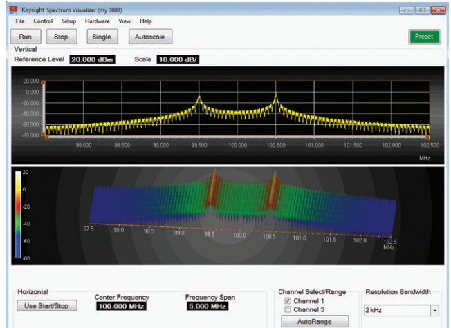
그림 40. ASV 스펙트로그램 측정에 대한 워터폴 보기
