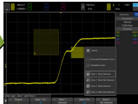
그림 15. 이상 신호를 발견하면 구역 박스를 그리고 그 위에서 실행시키면 됩니다.
